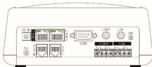
PBSP403/-SIP背面 (開発中)
